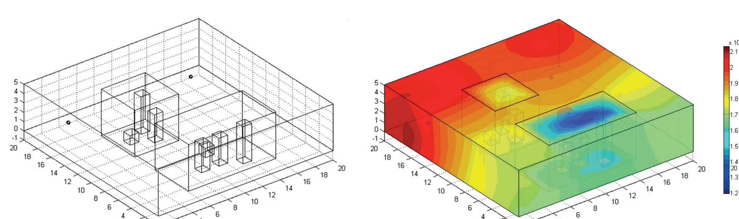
Simulation de la propagation acoustique dans un hall industriel intégrant deux sources sonores et deux zones d'encombrement. Résolution par éléments finis.
